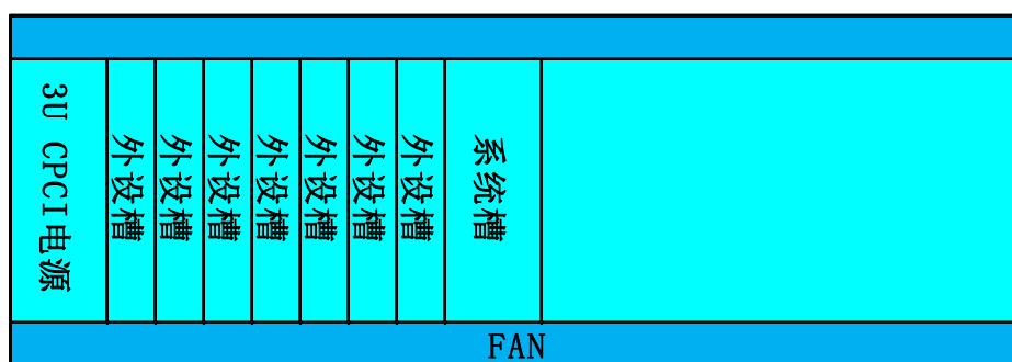
前视图
